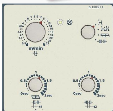
Панель управления MIRA 151 KGE
